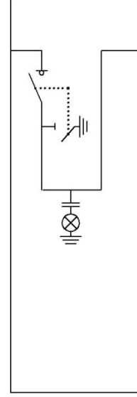
ŞEKİL - 9 YÜK AYIRICILI BARA BÖLME FONKSİYONEL BİRİMİ
