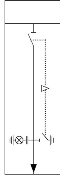
ŞEKİL - 6 AYIRICILI GİRİŞ-ÇIKIŞ FONKSİYONEL BİRİMİ
