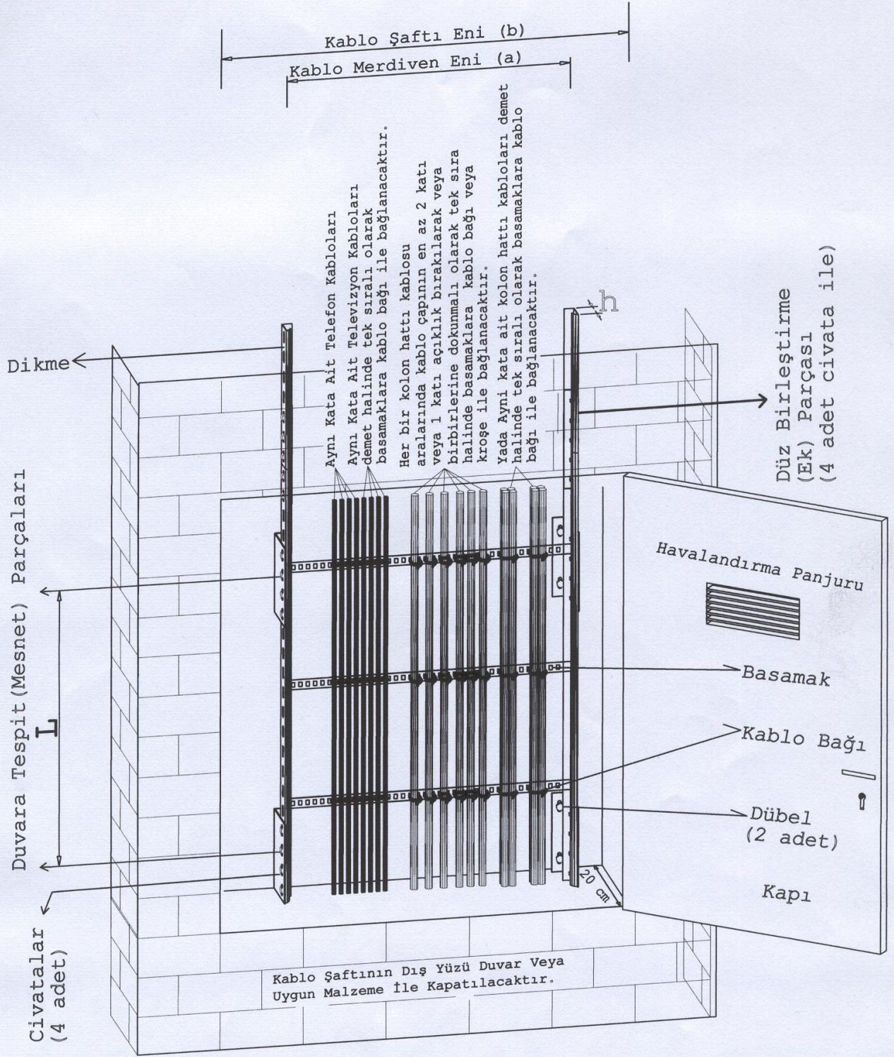
Şekil 1- Kablo Şaftı ve Örnek Kablo Merdiveni (Kablo Merdivenin Tek Parça Halinde Kablo Şaftı Arka Duvarına Monte Edilişi)
