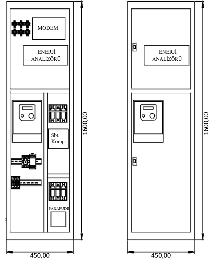
ÖLÇÜM VE KOMPANZASYON PANOSU
