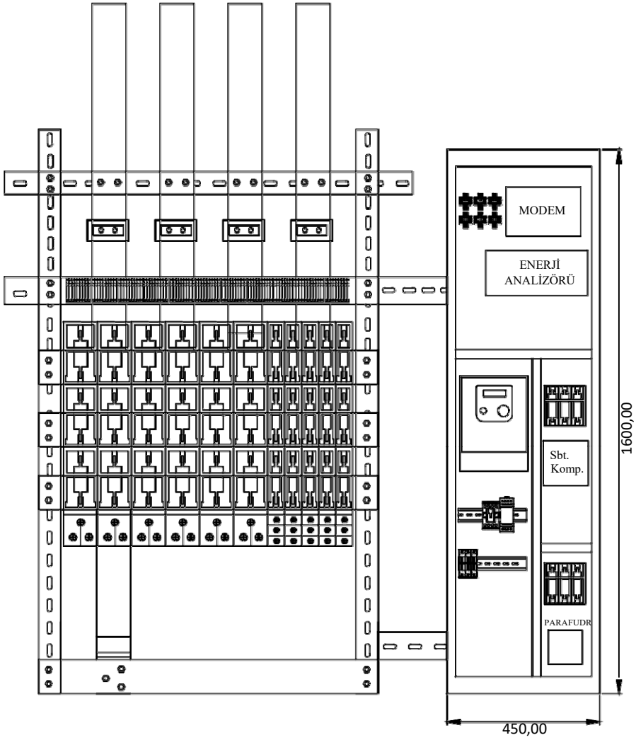
AG AÇIK BARA DÜZENİ
