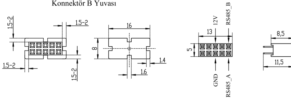
Konnektör B 2x5 pinli 2,54 mm V/T çift sıra dişi konnektör
