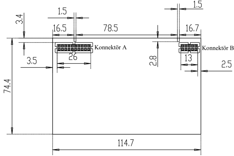
Modem Yuvası ve Konnektör Detayları
